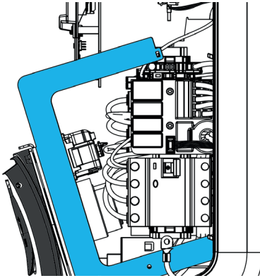
Image 5: Detachable subframe
